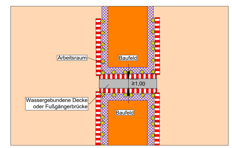
Detail: Wechselnde Fußgängerführung M= 1:250
